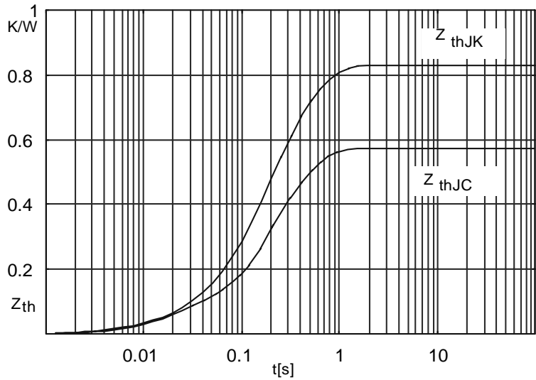
Transient thermal impedance per diode
