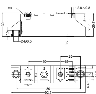
Fig. 38 (TO-240)
