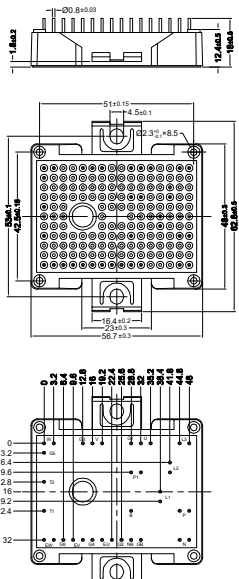
Fig. 70 (P2)
