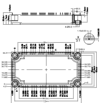
Fig. 68 (C7.3)
