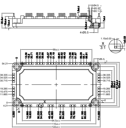
Fig. 64 (C7)
