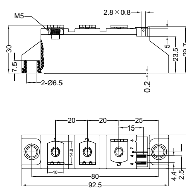
Fig. 36 (TO-240)
