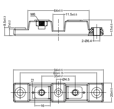
Fig. 44 (D2)
