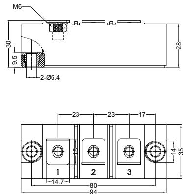
Fig. 3 (IAP)
