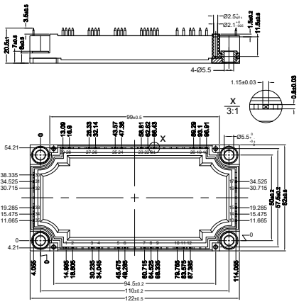
Fig. 65 (C7.1)
