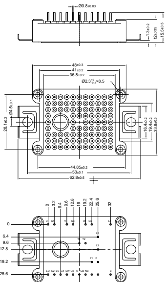
Fig. 69 (P1)
