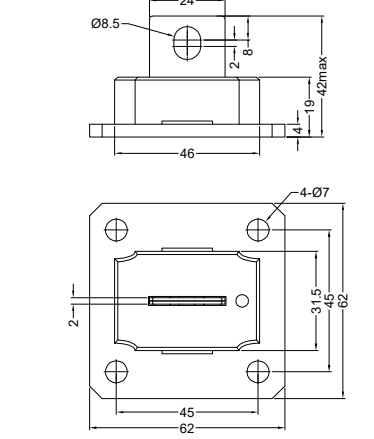
Fig.45 (D1)
