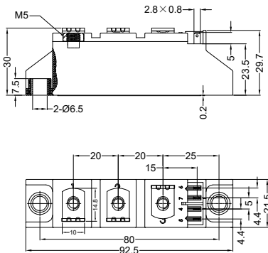
Fig. 31 (TO-240)
