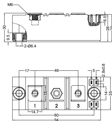
Fig. 4 (IAP)
