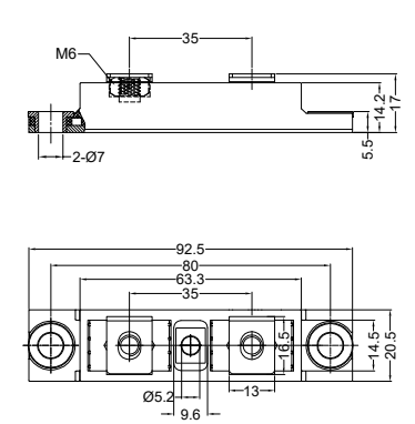
Fig.45 (D1)
