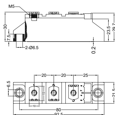
Fig. 33 (TO-240)
