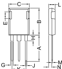
Fig. 54 (TO-247P)
