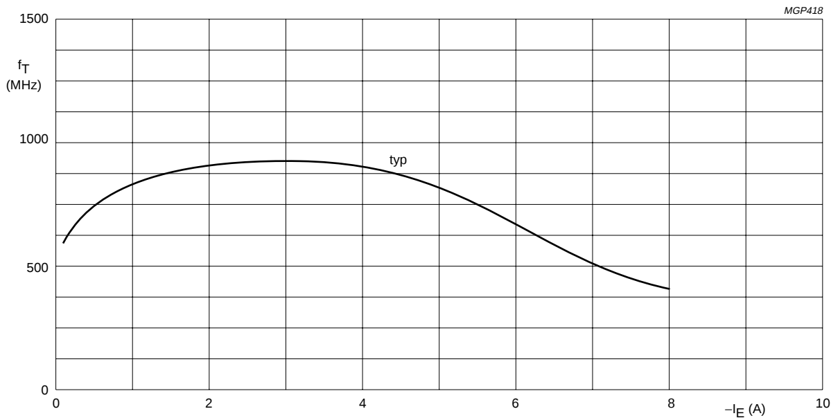
Fig.6 V_{CB} = 13,5\text{ V} ; f = 100\text{ MHz} ; T_j = 25^\circ\text{C} .
