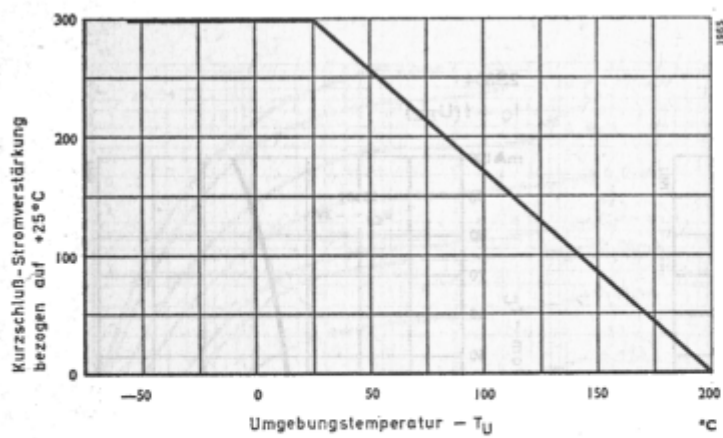
Typische Änderung von h_{21e} mit der Temperatur
