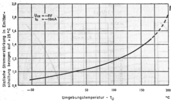
Typische Änderung von h_{FE} mit der Temperatur
