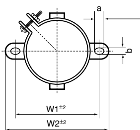
I type (øD = 51 to 90)
